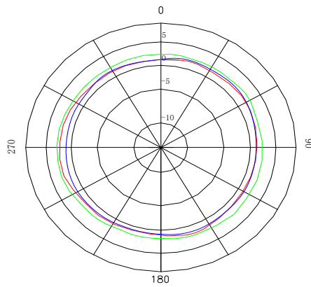
水平面方向图(2.4G天线) Horizontal Pattern
